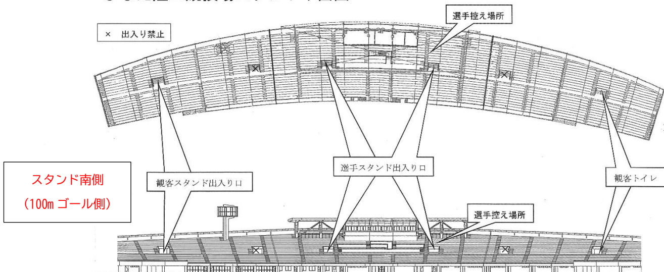
ひなた陸上競技場スタンド平面図
